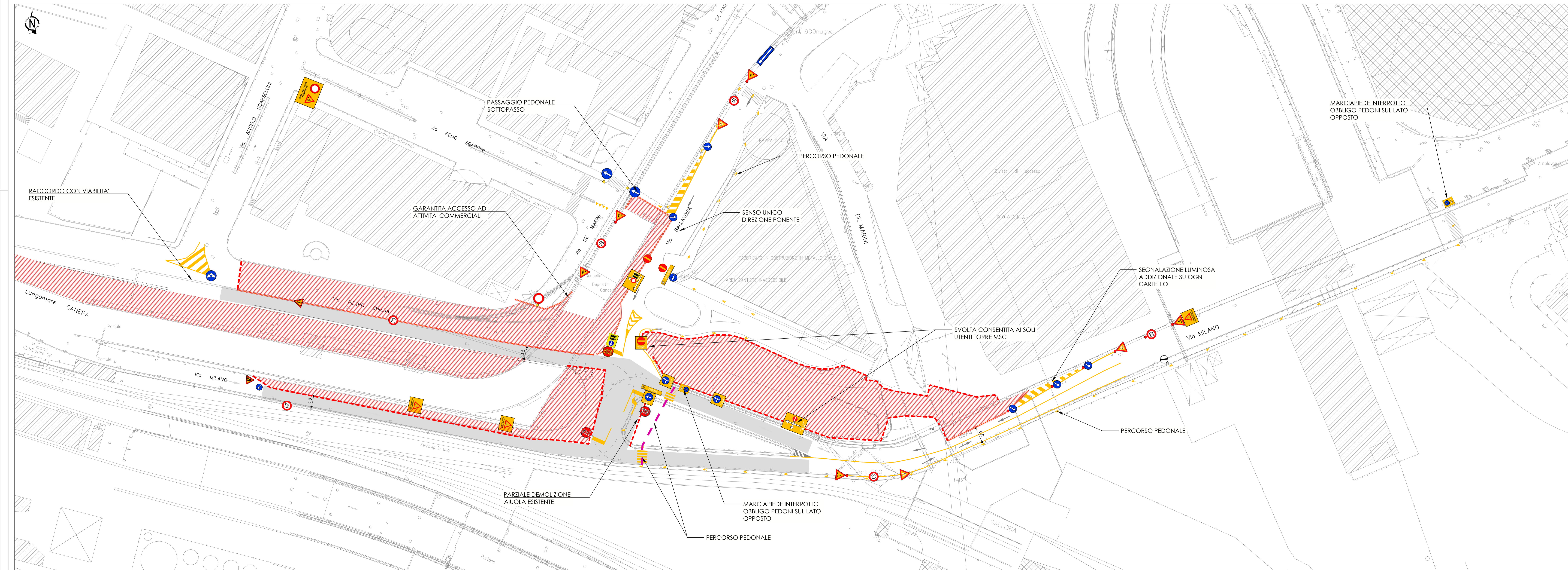
PLANIMETRIA CANTIERIZZAZIONE - scala 1:500
